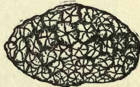
Truffles, ascoma
