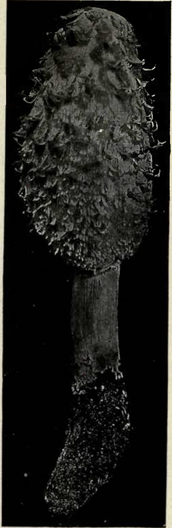
Coprinus comatus
