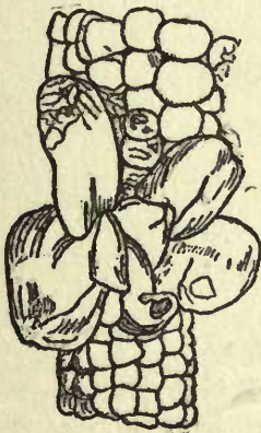
Corn smut
