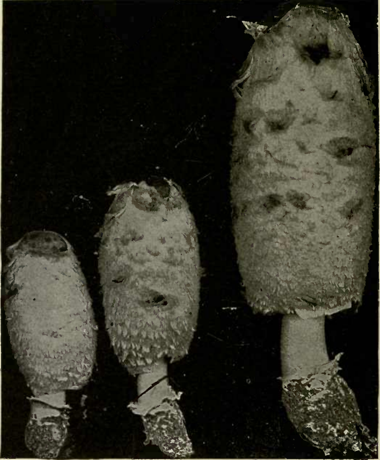
Coprinus comatus.
