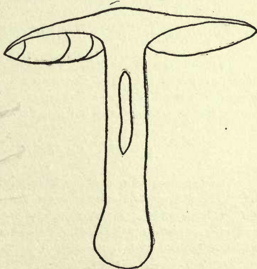
P. cervinus
