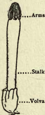
A. borealis
