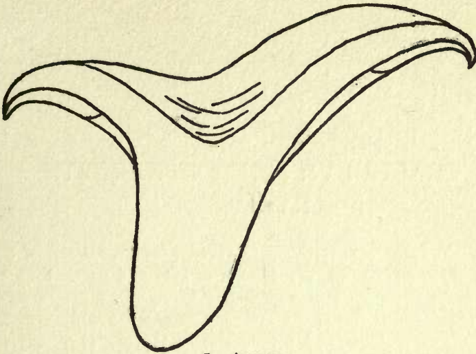
L. piberatus
